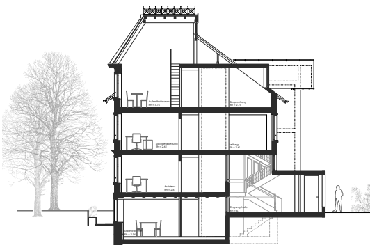
Querschnitt
