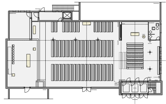
Grundriss Erdgeschoss nach Umbau
